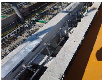
配力筋設置状況
