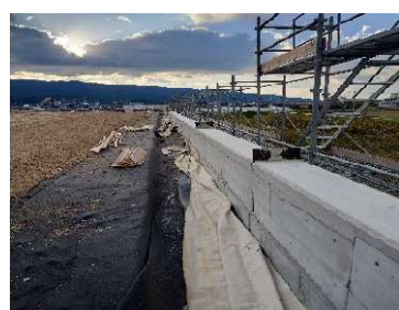
調整コンクリート打設
